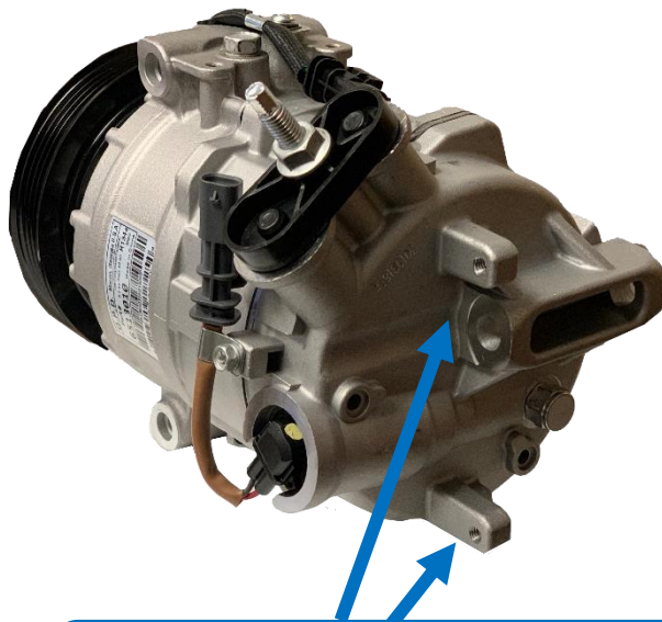
6513010 con agujeros para pernos de montaje del equipo original para el escudo térmico
